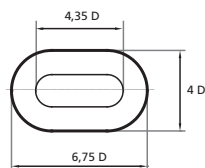
END LINK
