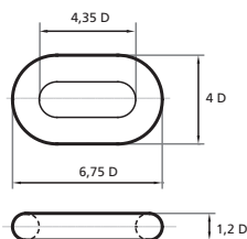
END LINK
