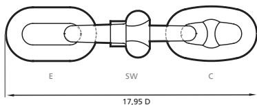
END LINK
